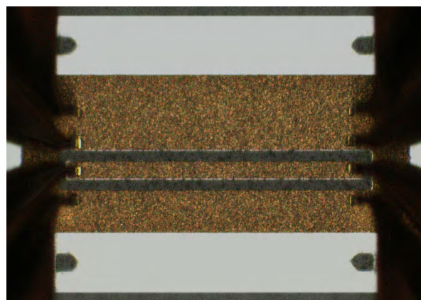
2つの向かい合ったGSSG TITAN™デュアルプローブを10μmの垂直オフセットトラベルでThru (Adj Gnd)標準器に触れた後、プローブを離れた時の写真。
