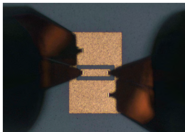
向かい合った2本のGS/GS TITAN™プローブをThru 標準器に接触させ、10μmの垂直オーバーラップした後、分離した状態
