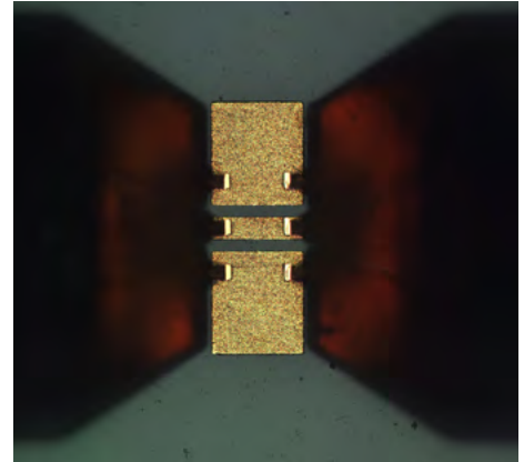
T110A-GSG100 プローブ使用時のAC2-2のスルーにオーバートラベル10 \mu\text{m} でコンタクトしたときの写真
